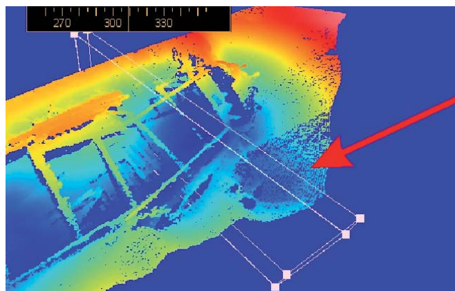
Obraz 3D rejonu wraka w dniu 17.10.2011 r. Obok wraka burdyny z XVIII wieku zalega wrak szkuty wiślanej (miejsce dziobnicy wskazuje strzałka).
