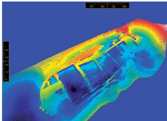
Zalegający w dnie Martwej Wisły wrak na obrazie z sondy wielowiązkowej – dobrze widoczny kształt dziobu, silne przechylenie na lewą burtę i oczyszczone z piasku ładownię
